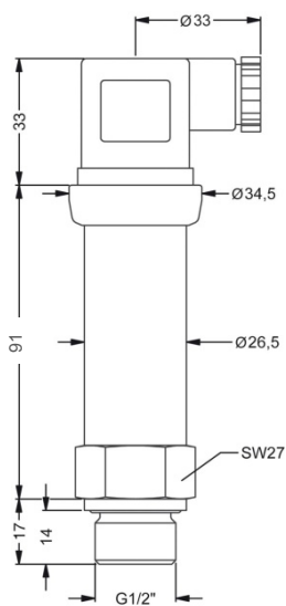
G1/2" DIN 3852
