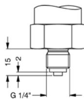
G1/4" EN 837
