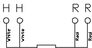
4-tråds koppling
