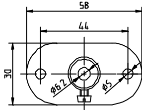
Konsole BR6.2
